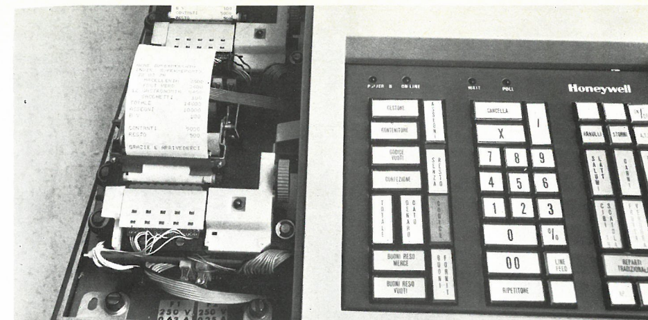
Figura 11: Particolare delle unità di stampa.
