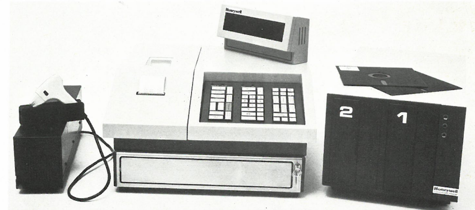
Figura 14: Il sistema P.O.S. basato su unità floppy disk con penna ottica O.C.R.
