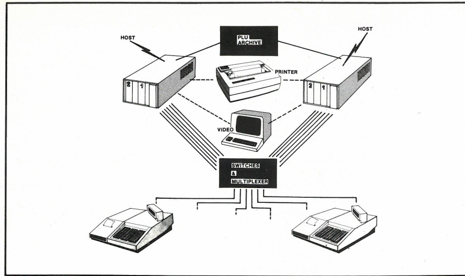
Figura 16: Il sistema P.O.S. basato su unità floppy disk in una configurazione doppia.
