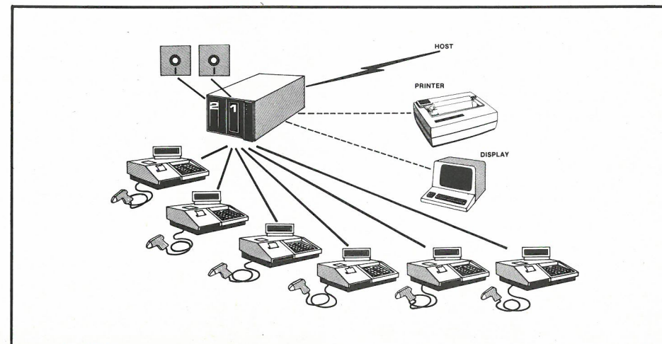
Figura 15: Schema di un sistema P.O.S. basato su unità floppy disk.
