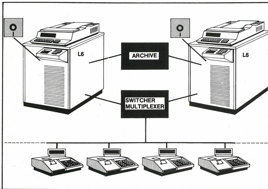
Figura 17: Il sistema P.O.S. basato su minielaboratori in una configurazione doppia.
